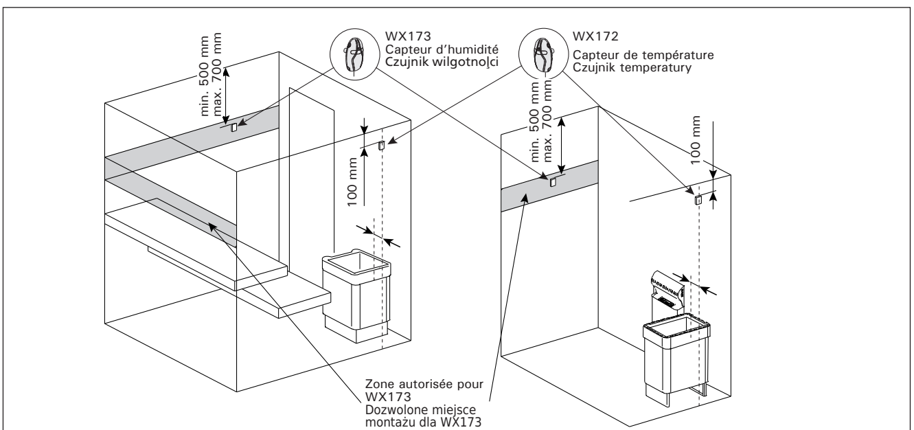
Figure 7. Emplacement des capteurs de température et d'humidité par rapport aux poêles en installation au sol Rysunek 7. Umiejscowienie czujników temperatury i wilgotności względem pieców podłogowych
