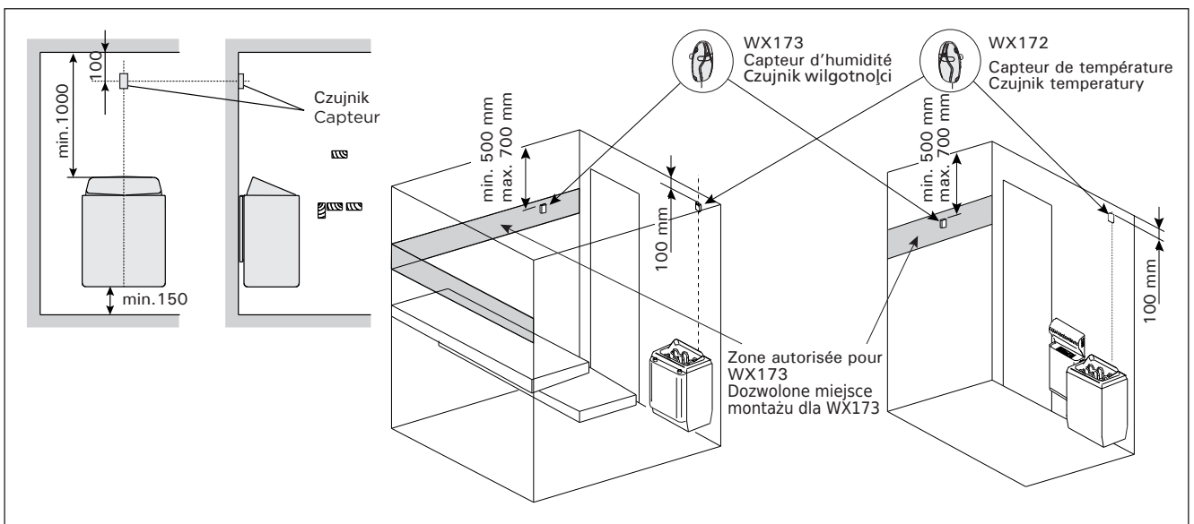
Figure 6. Emplacement des capteurs de température et d'humidité par rapport aux poêles en installation murale Rysunek 6. Umiejscowienie czujników temperatury i wilgotności względem pieców ściennych
